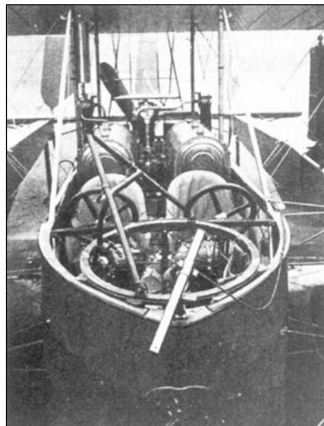
Slika 3: Detajli kabine Ca.33
