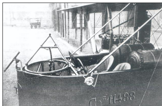
Slika 4: Detajli kabine Ca.33
